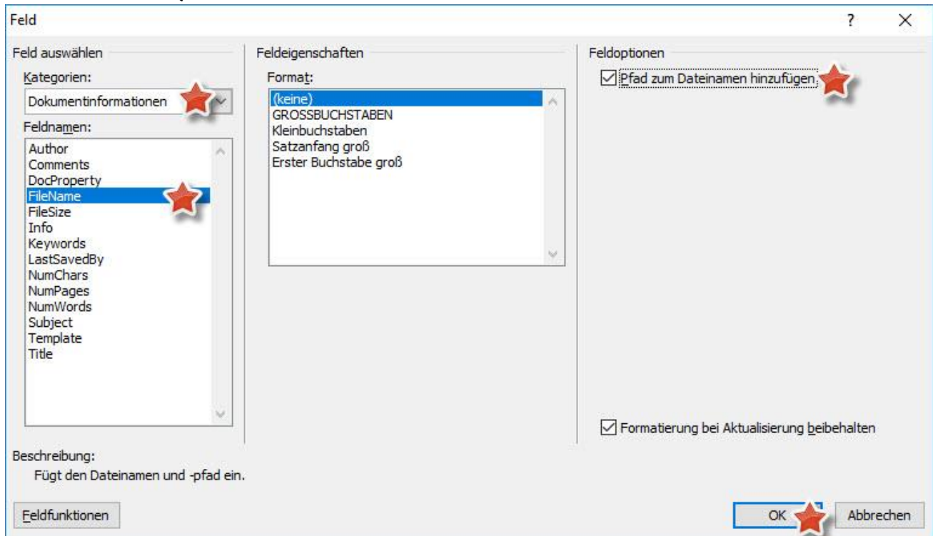
Abbildung 2: Fenster "Feld"
