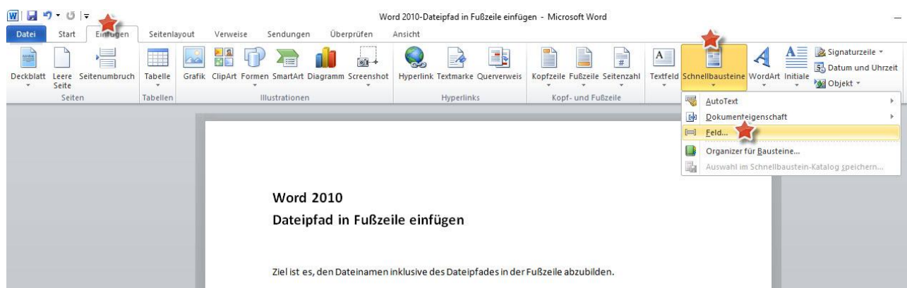
Abbildung 1: Schnellbausteine einfügen
